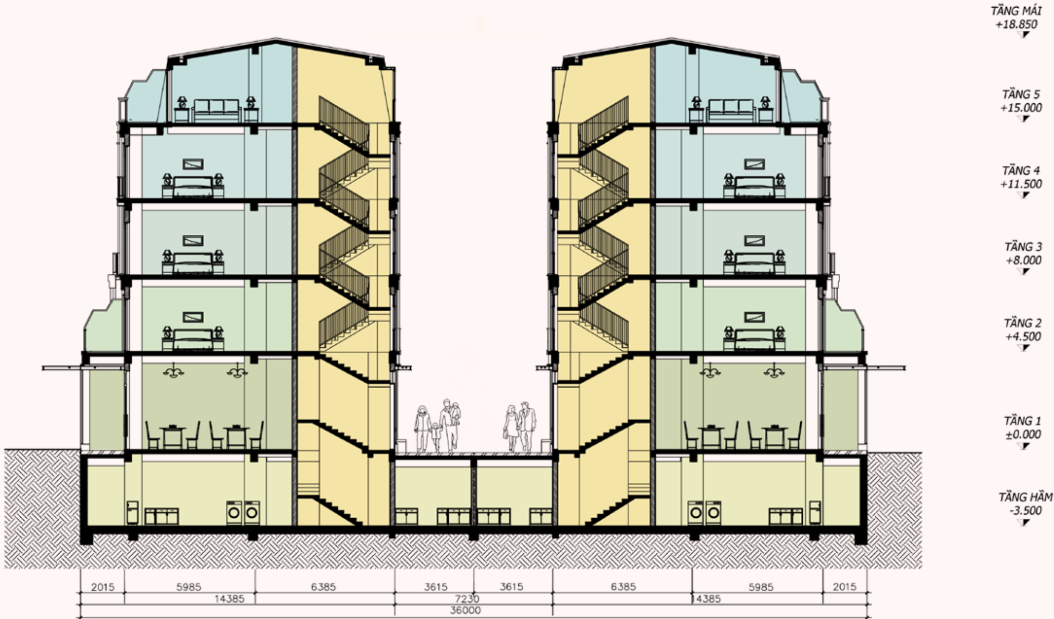
MẶT CẮT LÔ TMS 14
